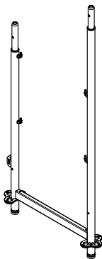
Základní rám EVB 67
